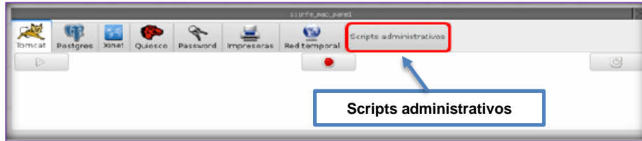
Imagen 7. Scripts administrativos
